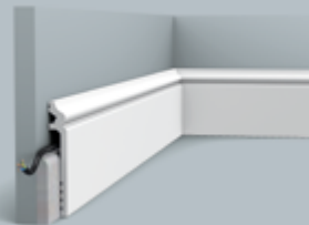
SX186 CONTOUR 200 x 13,8 x 2,2 cm Duropolymer ®
